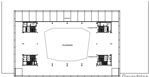
Grundriss
